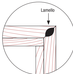
ASSEMBLAGE DU CADRE Tête et jambage
